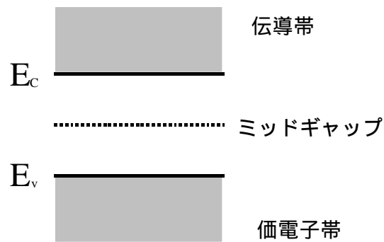
図1 エネルギーバンド図
